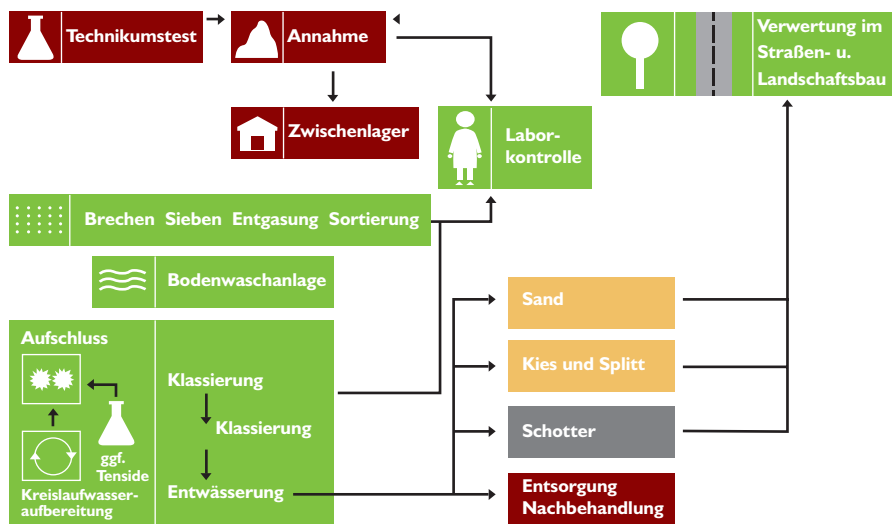
Schema des TERRALAVAR®-Verfahrens
